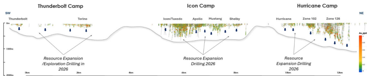
Figure 4 : coupe longitudinale orientée nord-est/sud-ouest traversant le projet Glenburgh, montrant la répartition des trous de forage et des résultats d'analyse, ainsi que l'émergence de trois camps bien délimités présentant une minéralisation quasi contiguë. Le camp Thunderbolt n'a pas encore fait l'objet de forages par Benz.
