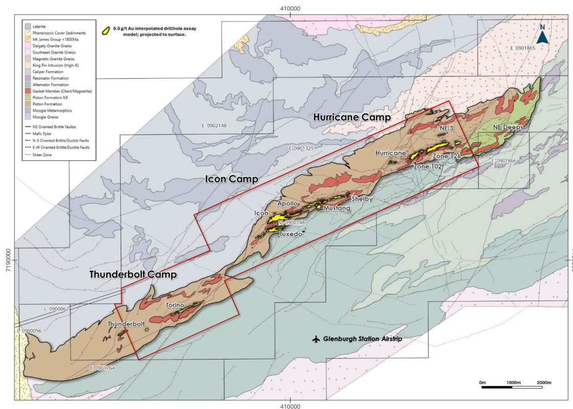
Figure 3 : camps aurifères de Glenburgh : interprétation géologique et structurale de Benz, superposée au modèle d'analyse des forages interpolé à 0,5 g/t Au, projeté en surface. Concession minière octroyée indiquée par un contour rouge.
